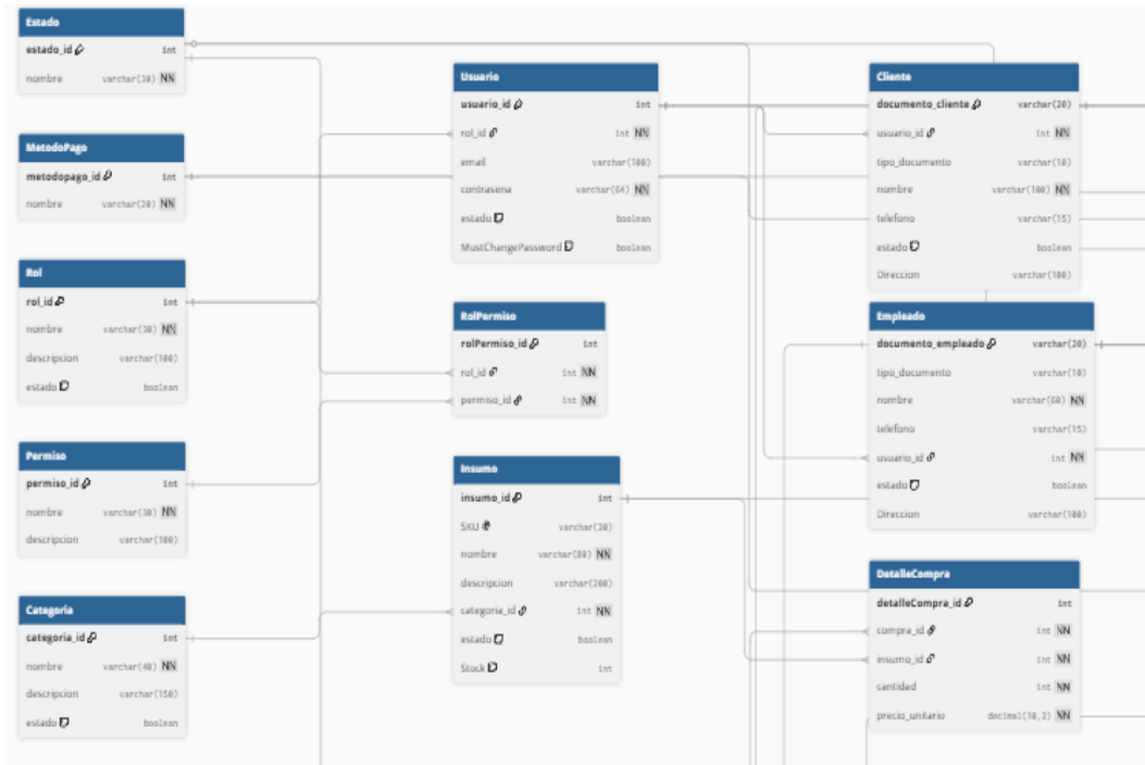
Figura 15. Modelo Relacional
